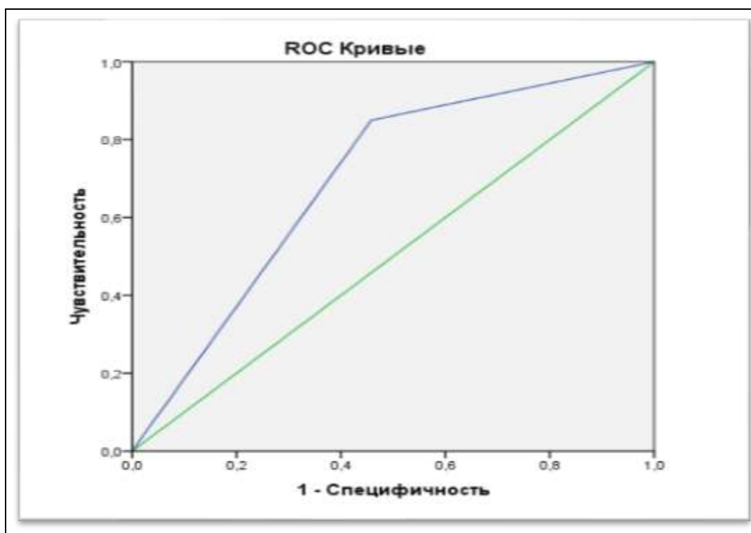
Рисунок 11 - ROC-кривая бинарной классификации приверженности по результатам ШП в наблюдательном исследовании АНТЕЙ
